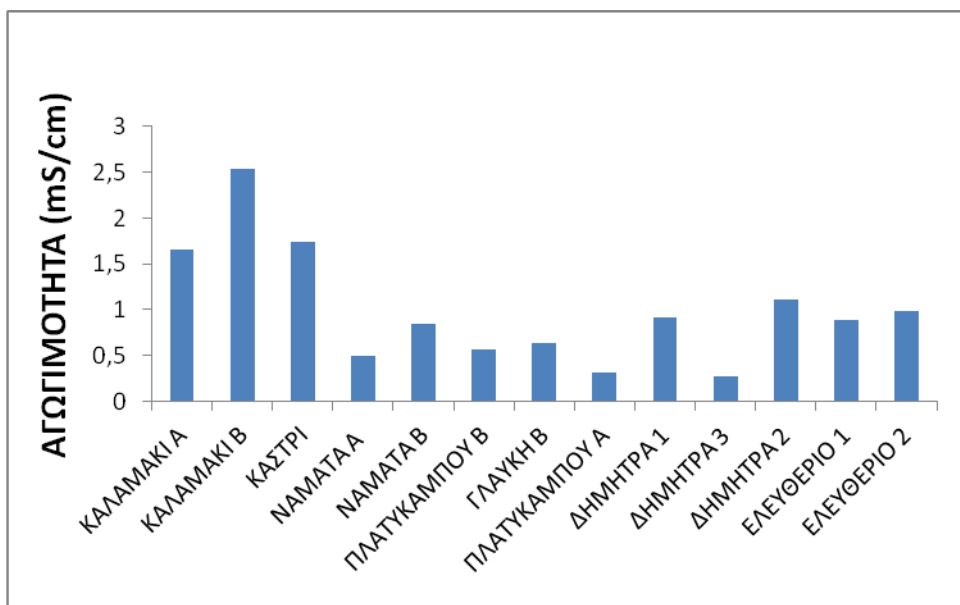
Εικόνα3.2.17 Διακύμανση Αγωγιμότητας στους μικρότερους ταμιευτήρες της Προστατευόμενης Περιοχής το Μάιο του 2012.
