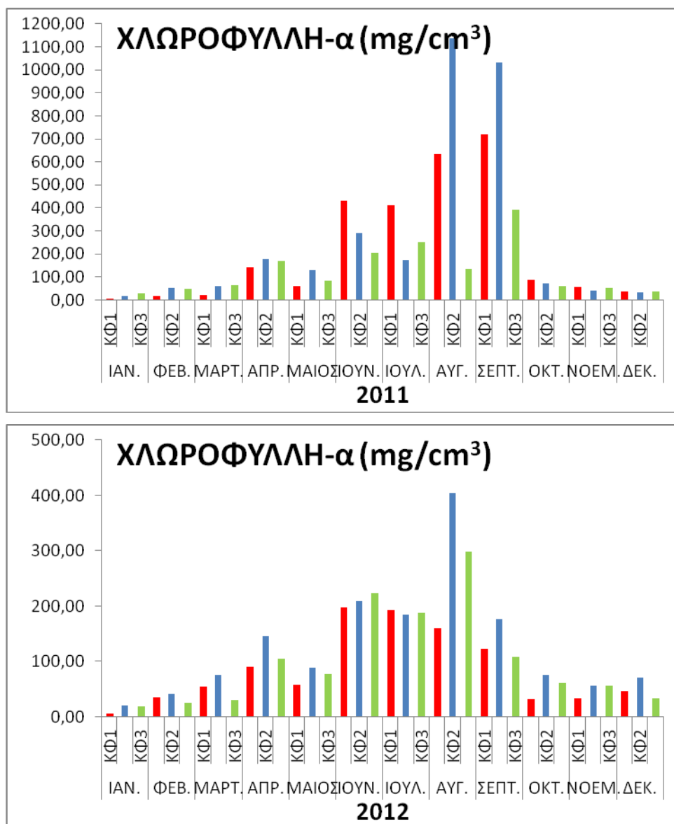
Εικόνα 3.2.9. Μηνιαία διακύμανση Χλωροφύλλης-α στη Λίμνη Κάρλα τα έτη 2011 και 2012.
