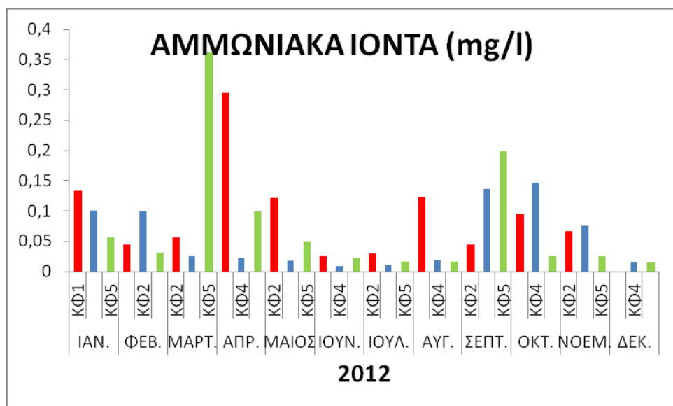
Εικόνα 3.2.7. Μηνιαία διακύμανση Αμμωνιακών ιόντων στη Λίμνη Κάρλα τα έτη 2011 και 2012.
