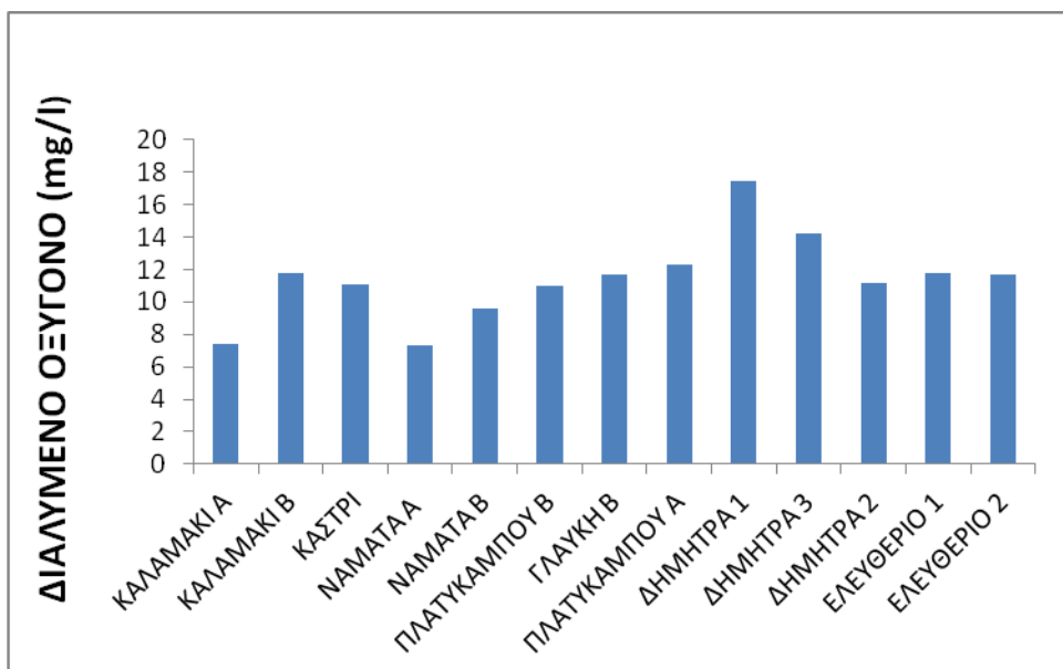
Εικόνα 3.2.15. Διακύμανση Διαλυμένου Οξυγόνου στους μικρότερους ταμιευτήρες της Προστατευόμενης Περιοχής το Μάιο του 2012.
