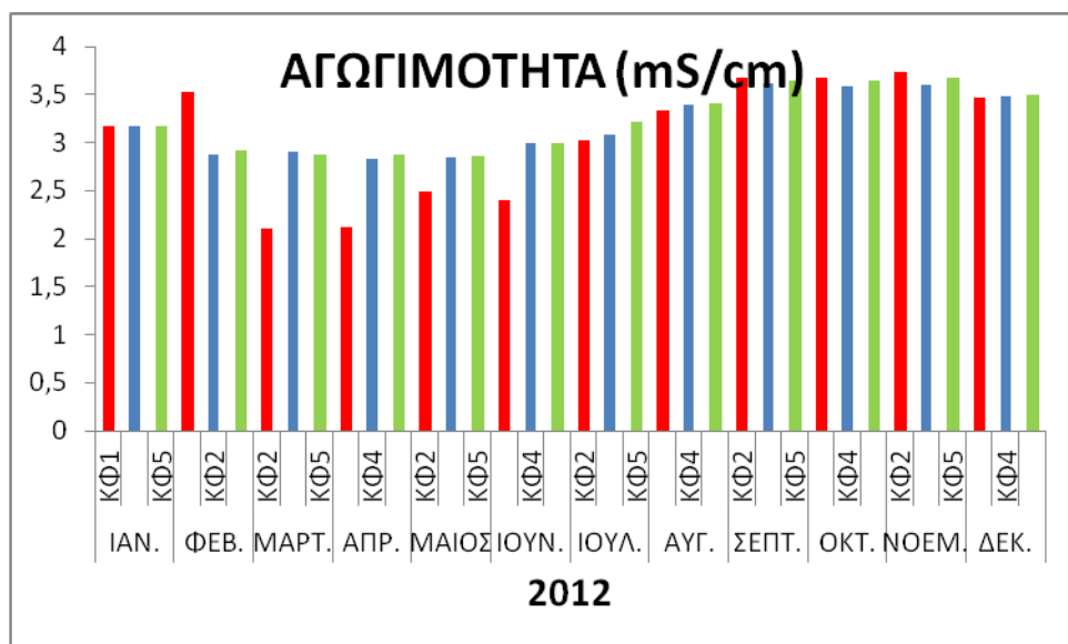
Εικόνα 3.2.5. Μηνιαία διακύμανση Αγωγιμότητας στη Λίμνη Κάρλα τα έτη 2011 και 2012.
