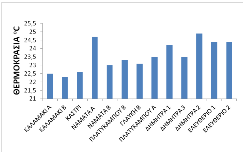
Εικόνα 3.2.16. Διακύμανση Θερμοκρασίας στους μικρότερους ταμιευτήρες της Προστατευόμενης Περιοχής το Μάιο του 2012.
