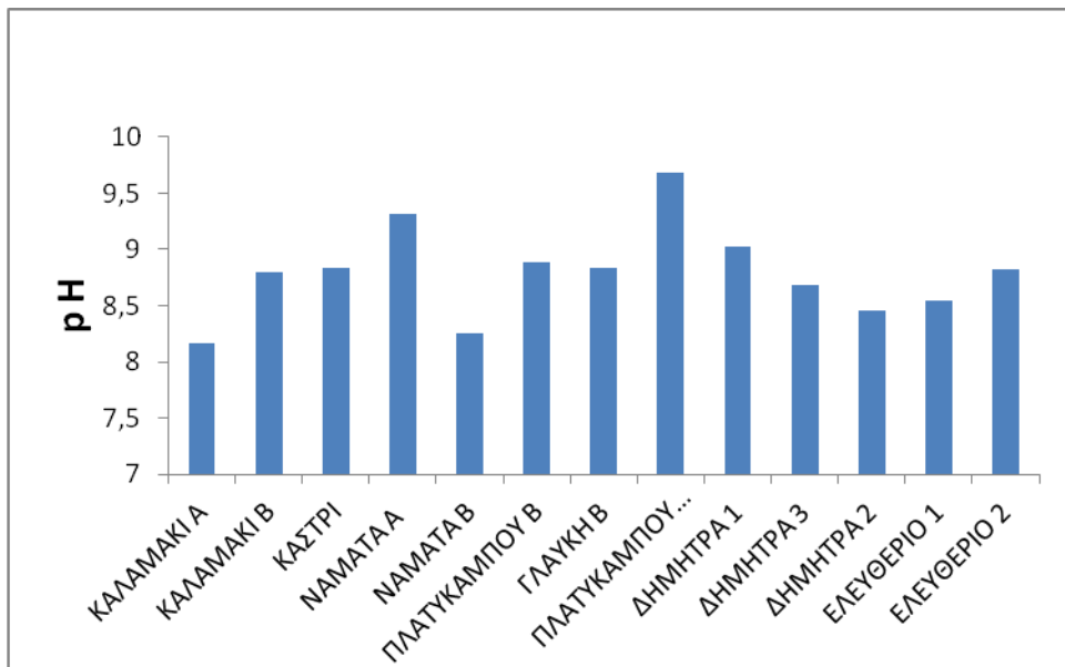
Εικόνα 3.2.14. Διακύμανση pH στους μικρότερους ταμιευτήρες της Προστατευόμενης Περιοχής το Μάιο του 2012.
