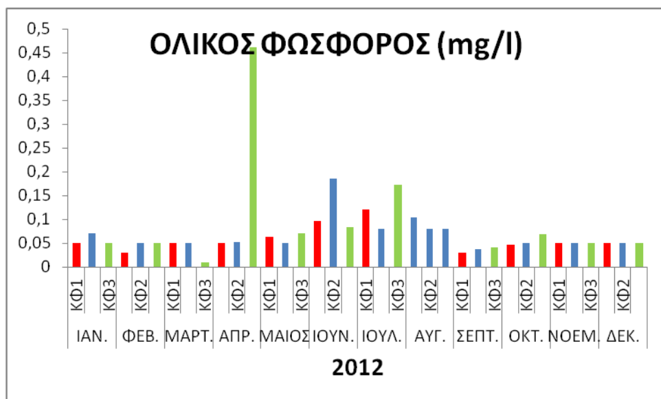
Εικόνα 3.2.8. Μηνιαία διακύμανση Φωσφορικών ιόντων και Ολικού Φωσφόρου στη Λίμνη Κάρλα τα έτη 2011 και 2012.
