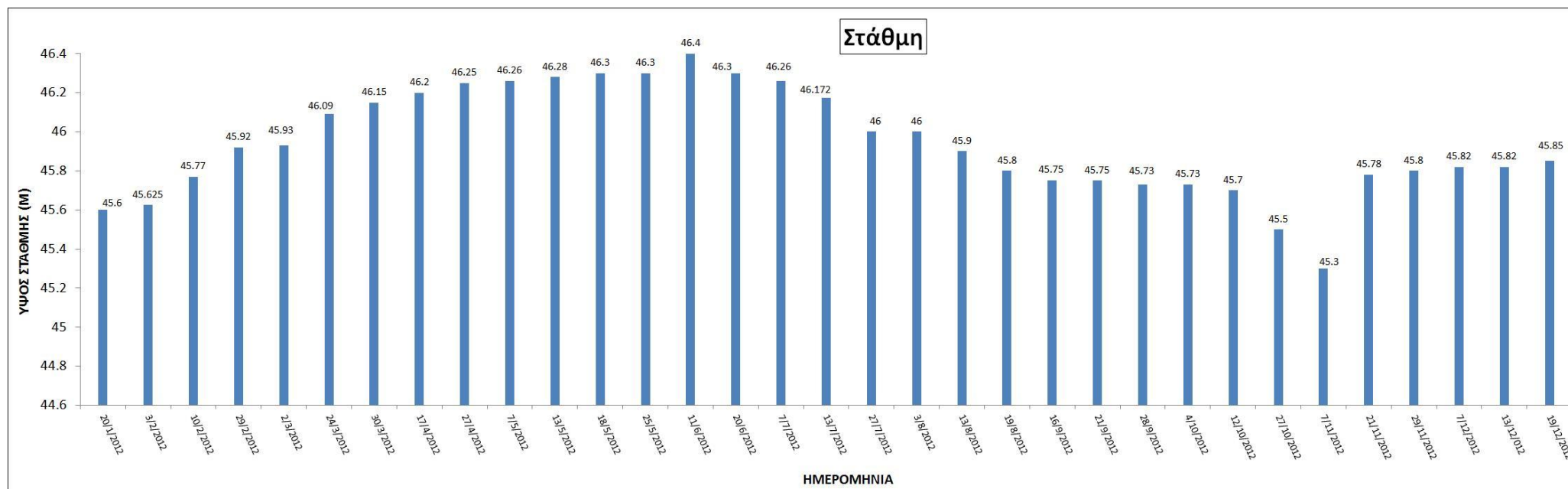
Εκόνα 2.1.2. Γραφική απεικόνιση της χρονοσειράς της στάθμης της λίμνης για το έτος 2012.
