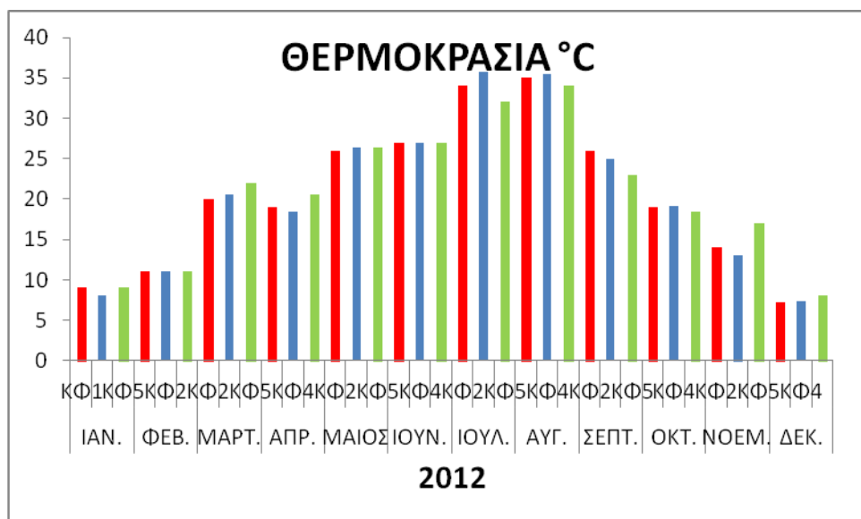
Εικόνα 3.2.4. Μηνιαία διακύμανση Θερμοκρασίας στη Λίμνη Κάρλα τα έτη 2011 και 2012.
